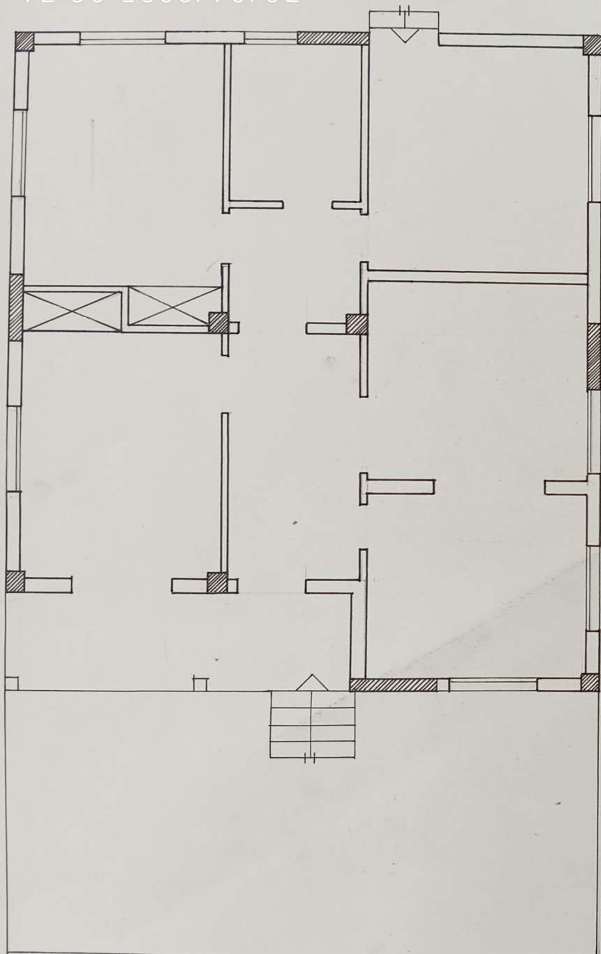
ΚΑΤΟΨΗ ΑΠΟΤΥΠΩΣΗΣ
