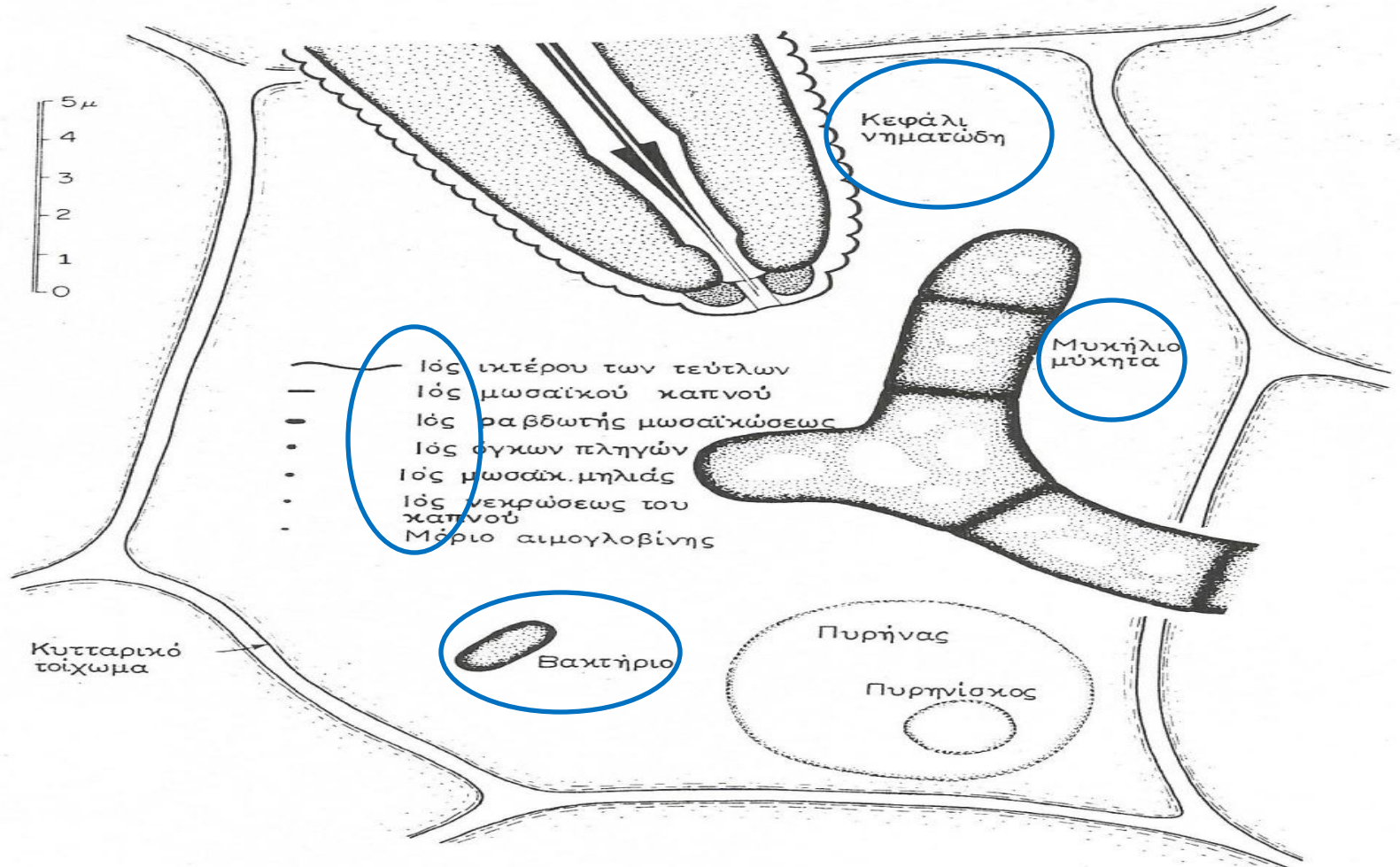
Σχ. 3.1. Διάγραμμα του σχήματος και του μεγέθους ορισμένων φυτοπαθογόνων σε σχέση με το φυτικό κύτταρο.
